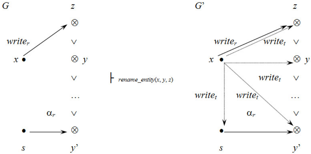
Рис. 18. Пример применения правила rename\_entity(x, y, z)
